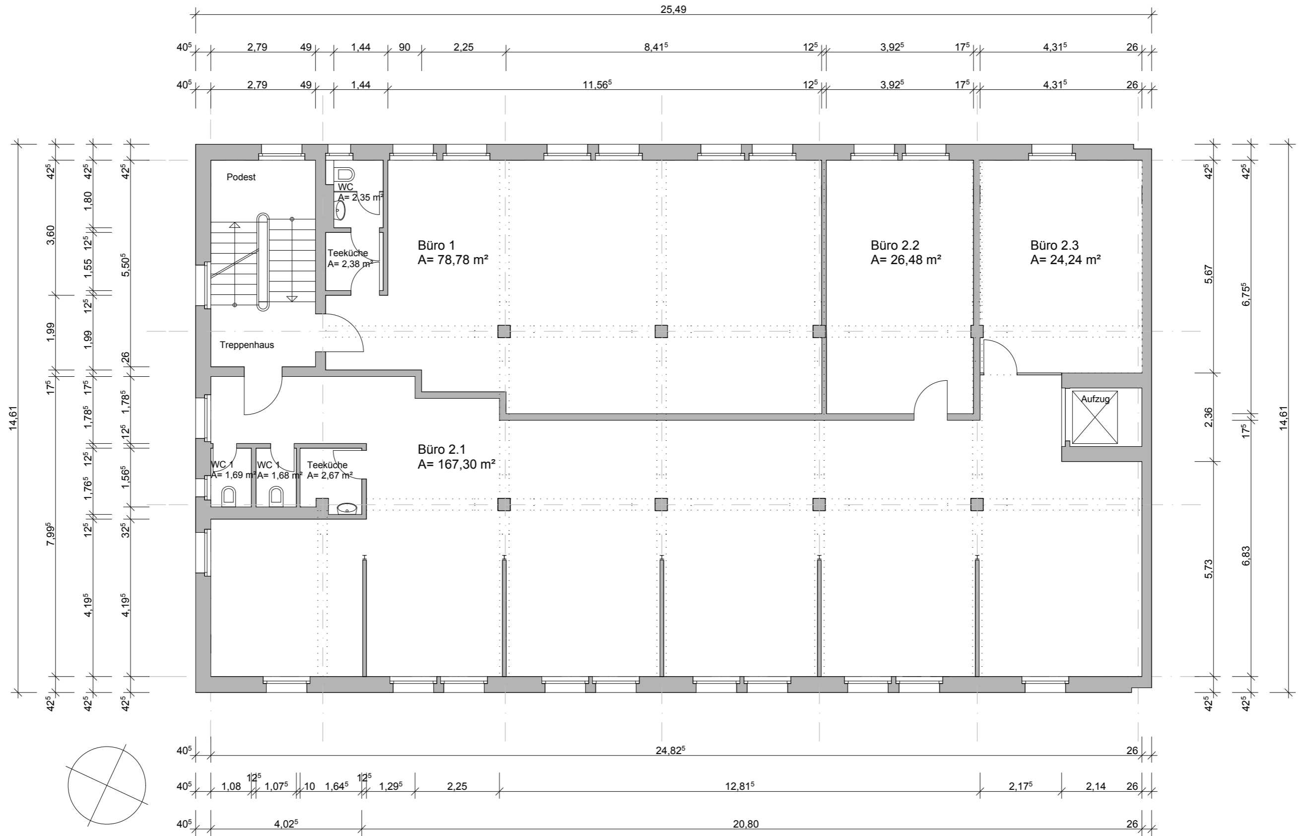
Grundriss 2. Obergeschoss
